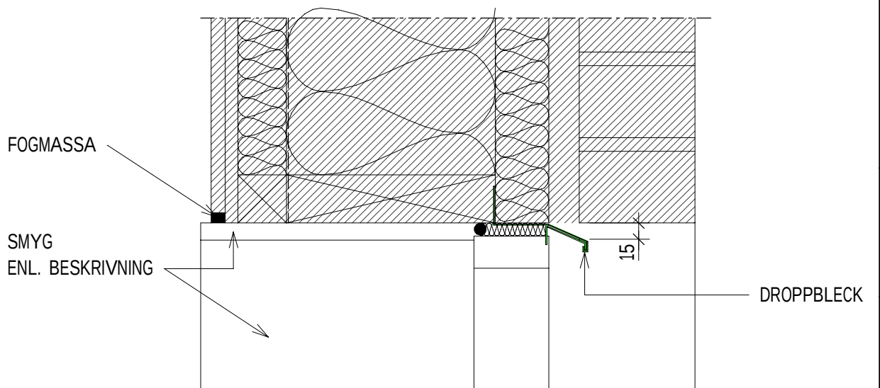
VD16 PRINCIPDETALJ 1:5 METALLPARTI
