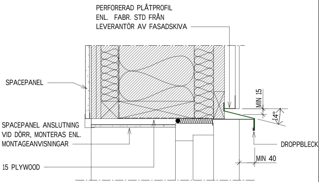
VD15 PRINCIPDETALJ 1:5 STÅLDÖRR
