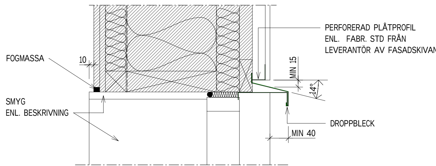
VD13 PRINCIPDETALJ 1:5 METALLPARTI
