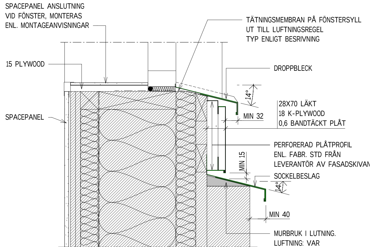
VD5 PRINCIPDETALJ 1:5 FÖNSTER HÖJD TEGELSOCKEL I LIV MED HÖJD DET VD3
