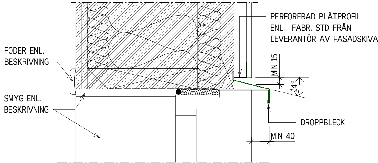
VD6 PRINCIPDETALJ 1:5 STÅLDÖRR
