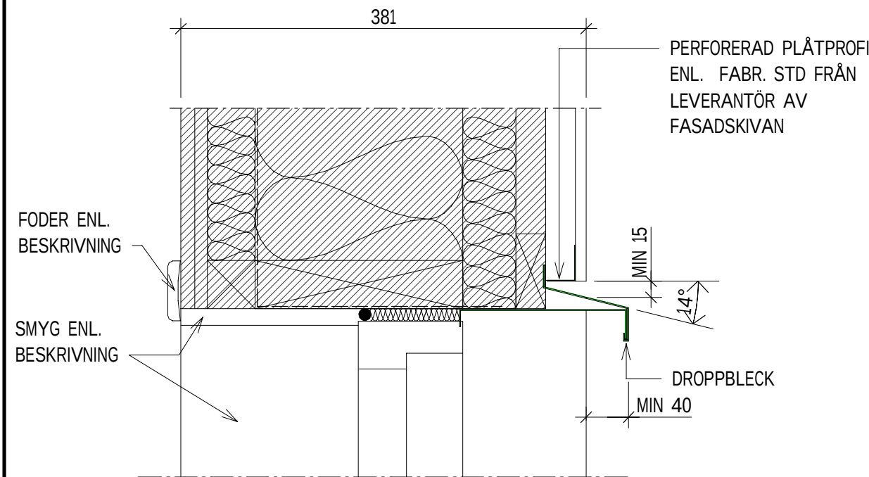
VD8 PRINCIPDETALJ 1:5 DÖRR FLÅKTRUM PLAN 2
