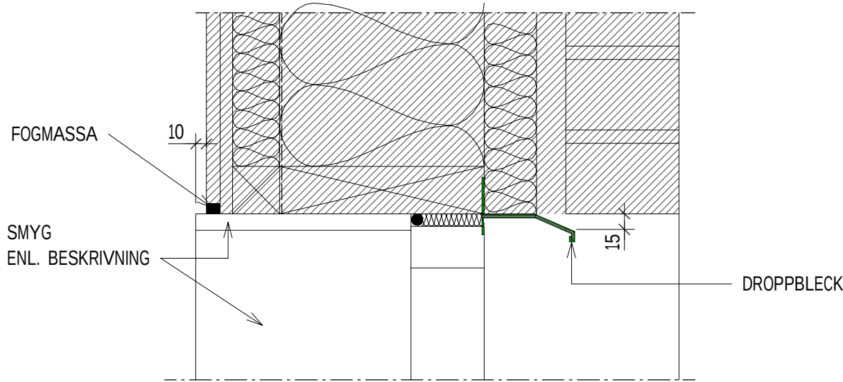
VD2 PRINCIPDETALJ 1:5 FÖNSTER
