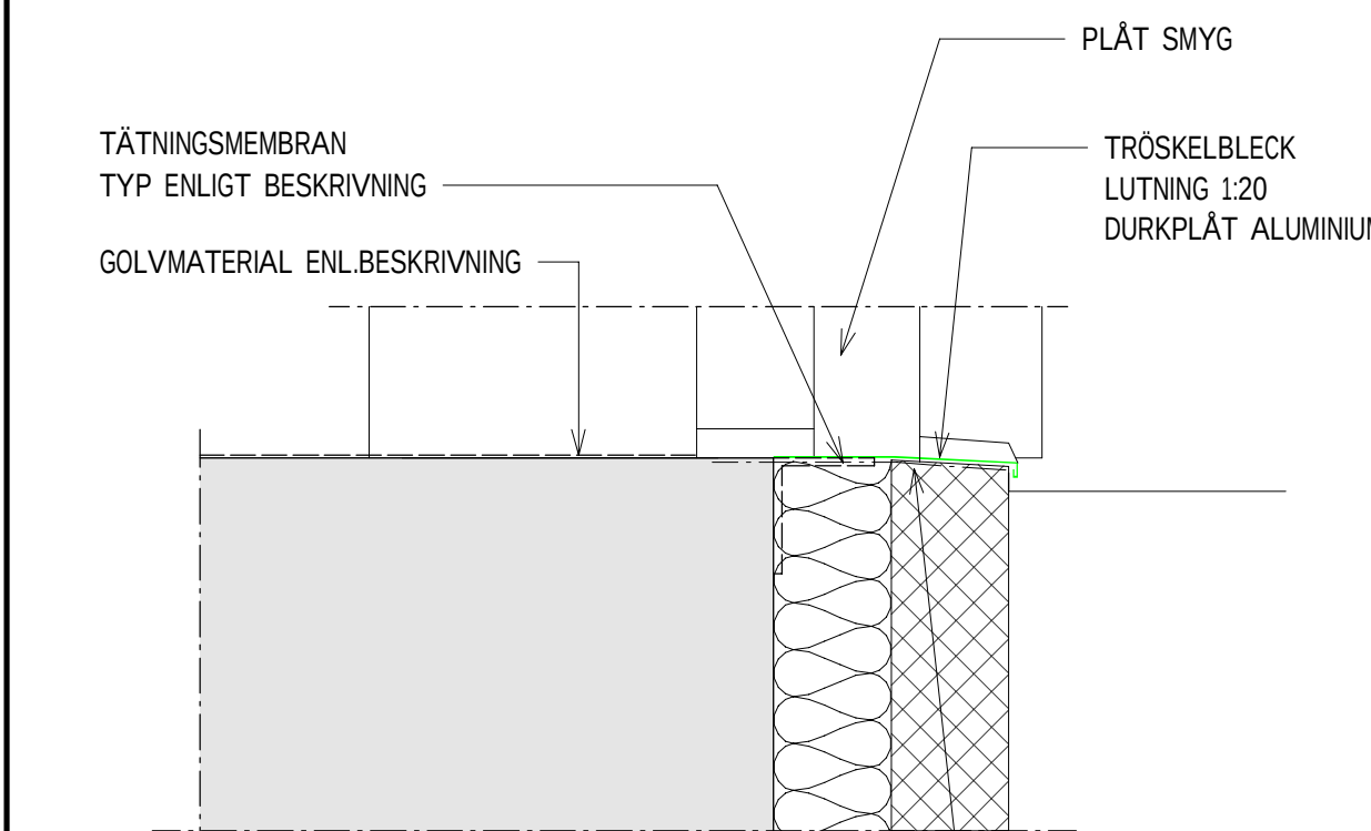
VD10 PRINCIPDETALJ 1:5 METALLPARTI
