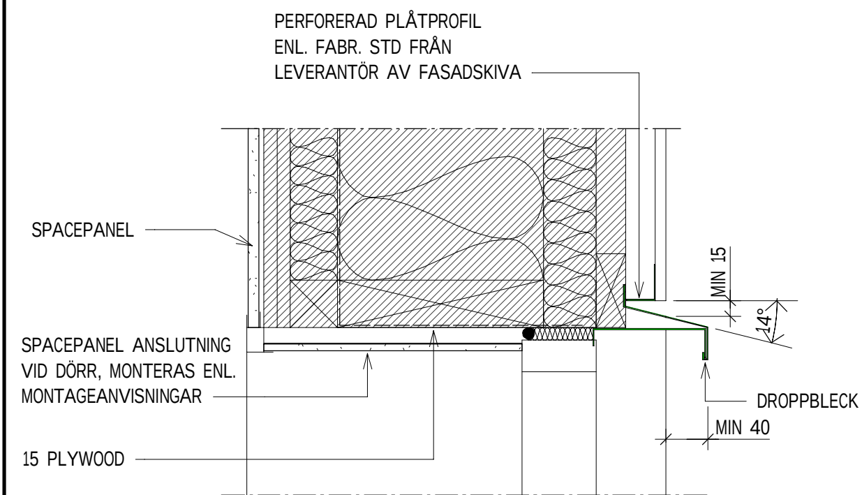
VD9 PRINCIPDETALJ 1:5 METALLPARTI
