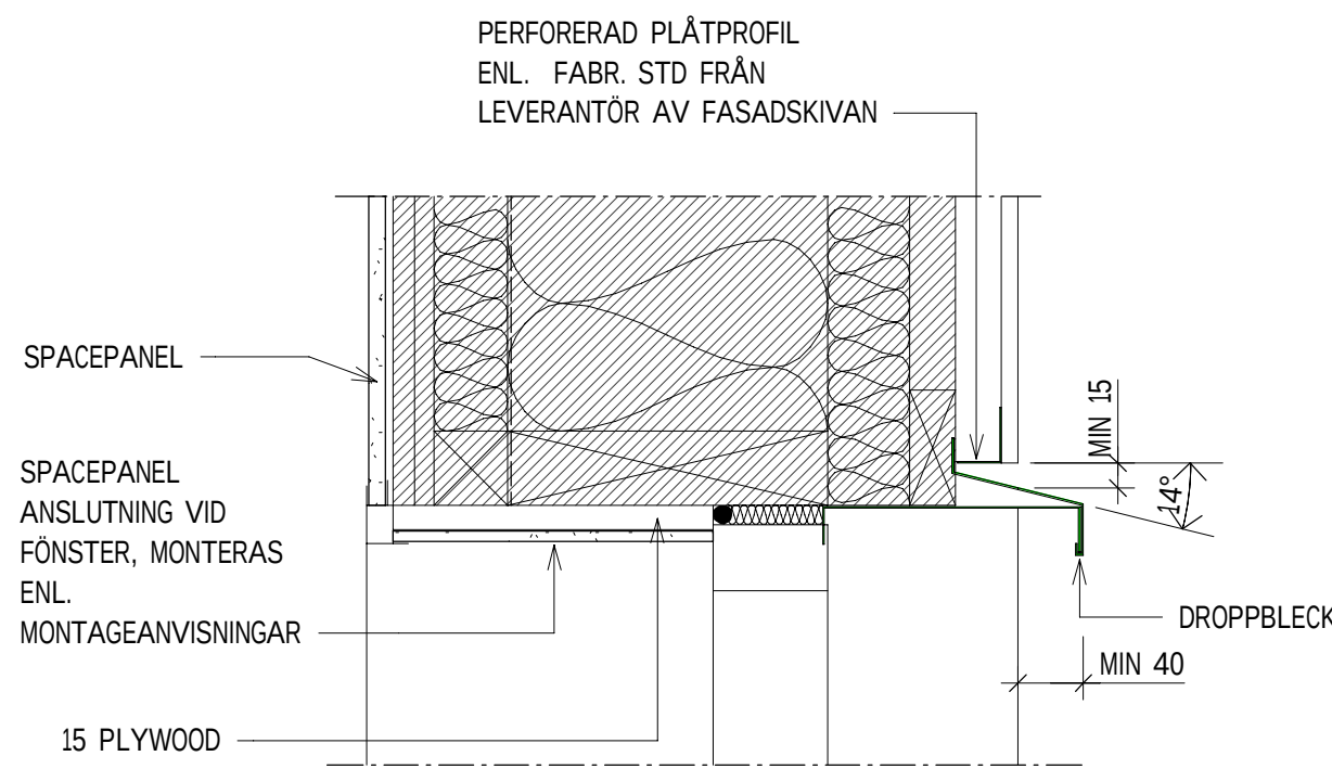
VD11 PRINCIPDETALJ 1:5 FÖNSTER
