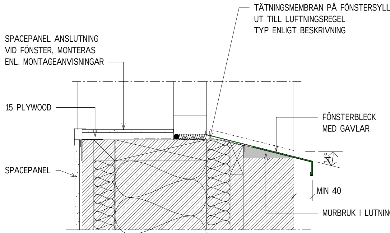
VD12 PRINCIPDETALJ 1:5 FÖNSTER
