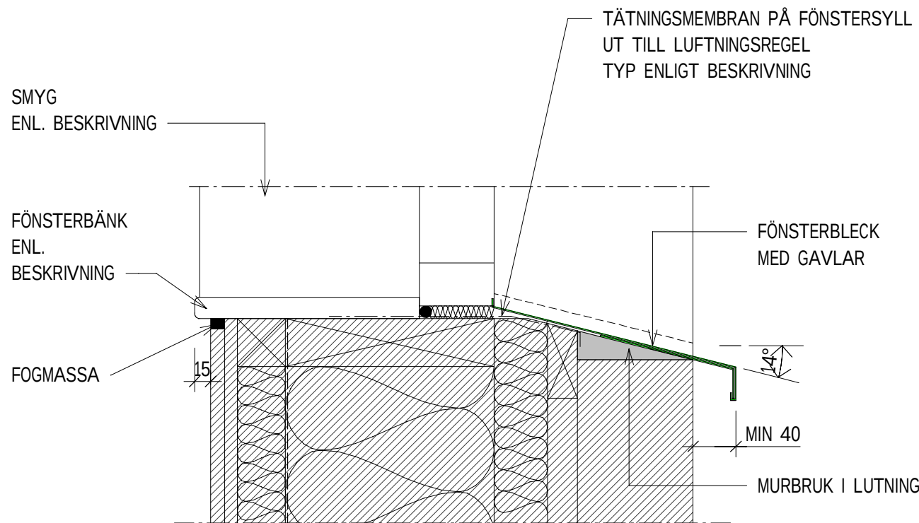
VD3 PRINCIPDETALJ 1:5 FÖNSTER
