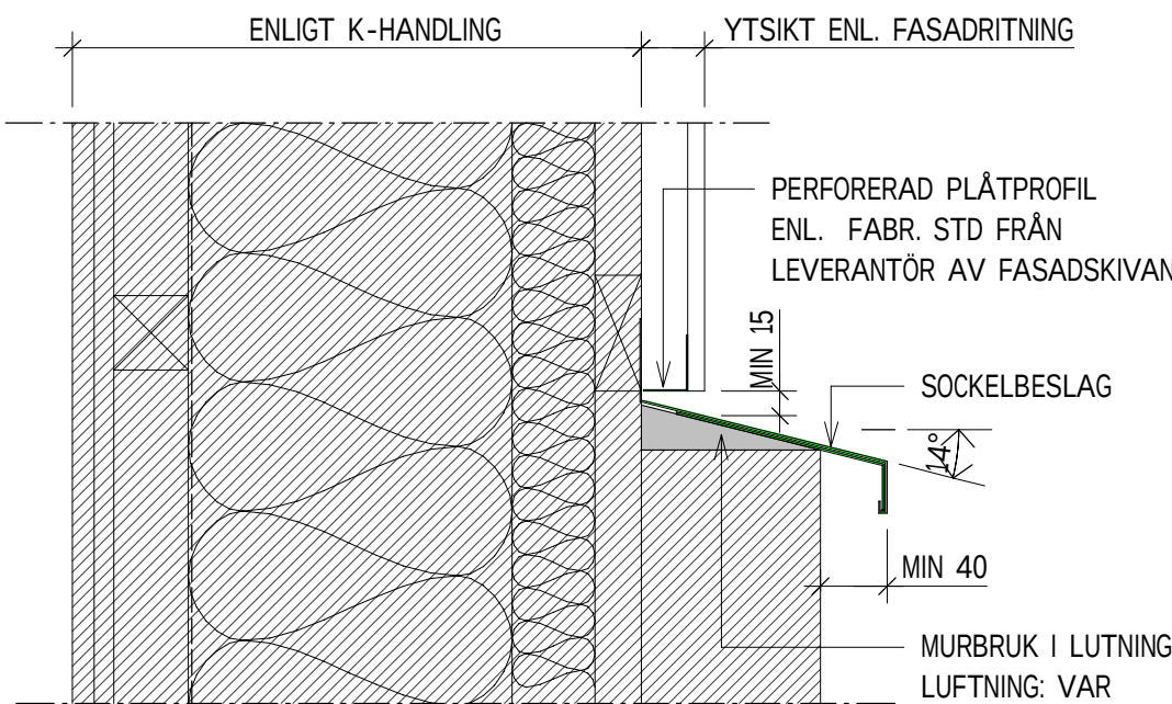
VD1 PRINCIPDETALJ 1:5 HÖJD TEGELSOCKEL I LIV MED HÖJD DET VD3
