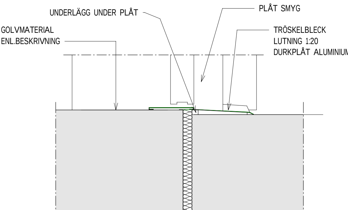
VD14 PRINCIPDETALJ 1:5 STÅLDÖRR SOPRUM
