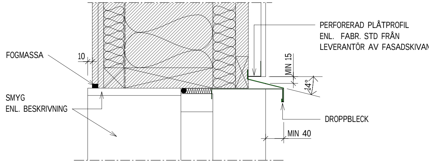
VD4 PRINCIPDETALJ 1:5 FÖNSTER
